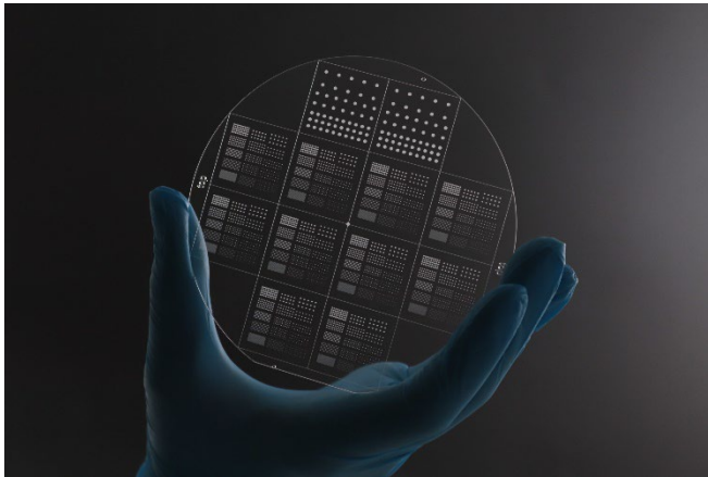
Bild 2: Mitarbeiter hält mikrostrukturierten Wafer in der Hand, der einzelne 22 x 22 mm Chips zeigt. Gut zu erkennen, die Mikrometer großen Wells ins Glas. © LPKF Laser & Electronics AG.
