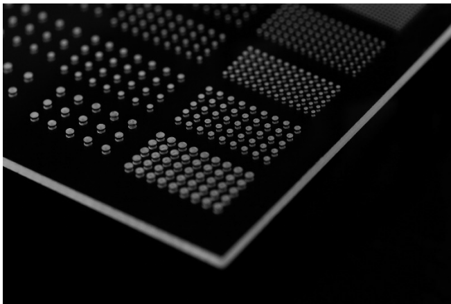
Bild 3: Einzelner Glas Chip mit Wells von mit 50 \mu\text{m} bis 400 \mu\text{m} Durchmesser. © LPKF Laser & Electronics AG.
